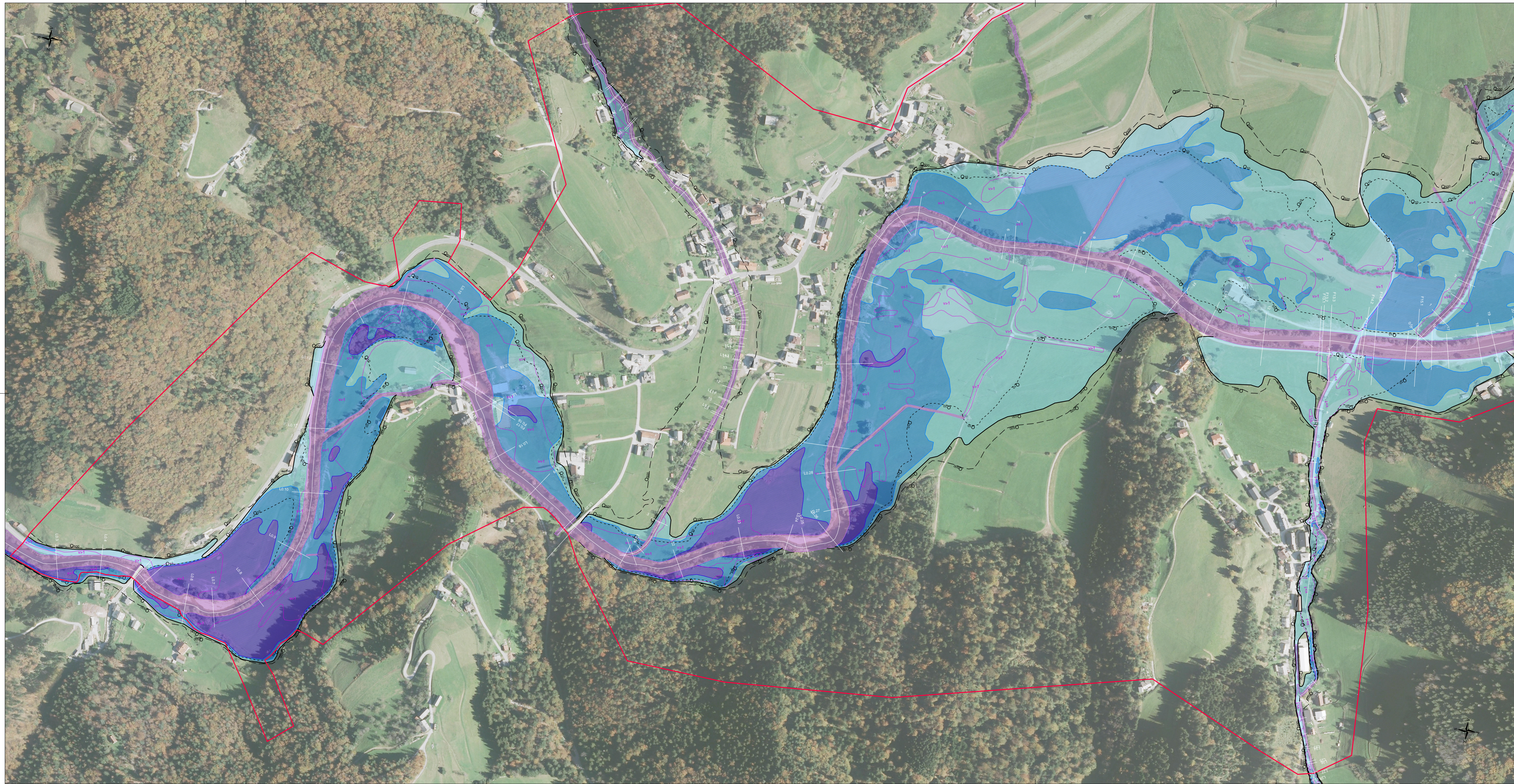
Karta poplavne nevarnosti - globine M 1:2000
